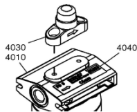
4030 - 1617 7048 00 Indicador Saturação
